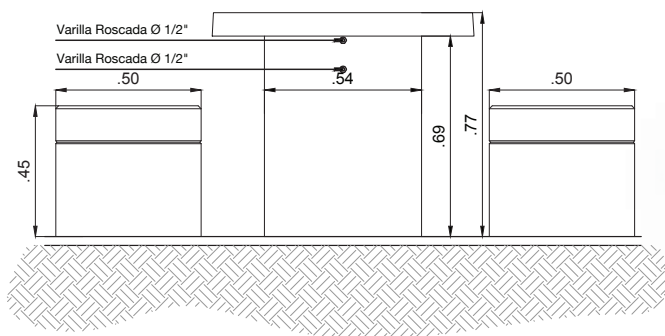
Vista Lateral
