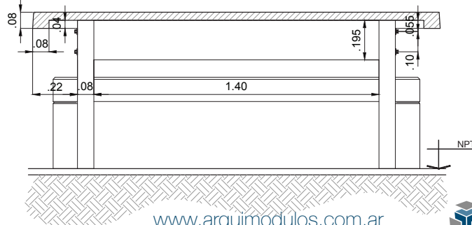
Corte Transversal
