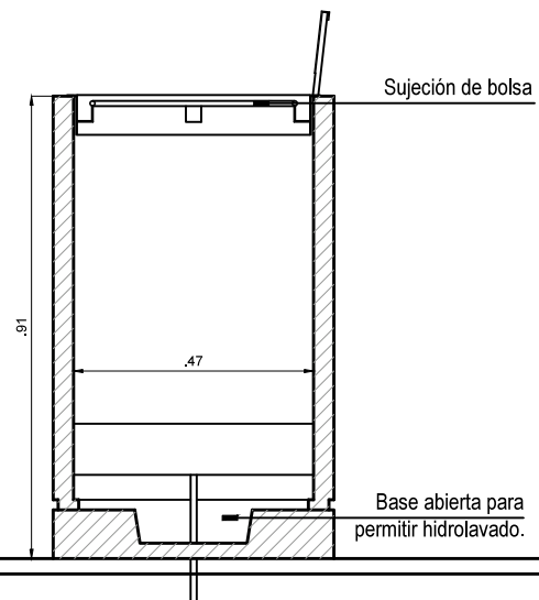
Corte Conjunto
