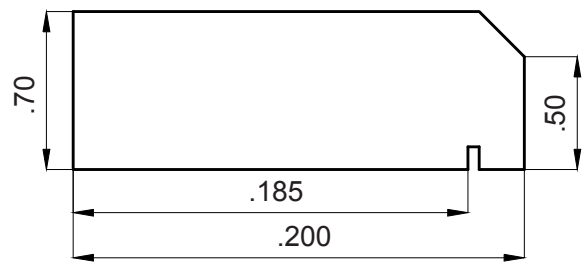
Vista Lateral
